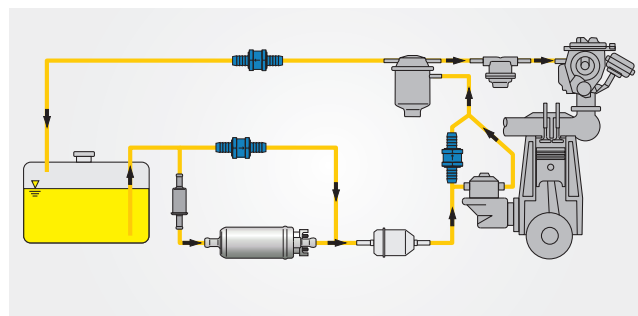
Пример применения: Карбюраторный двигатель с дополнительным подключаемым электрическим насосом
